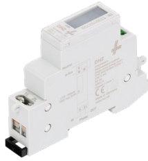
Meter 1f DHZ 5/63-M-BUS 1× 230 V, 63 A
